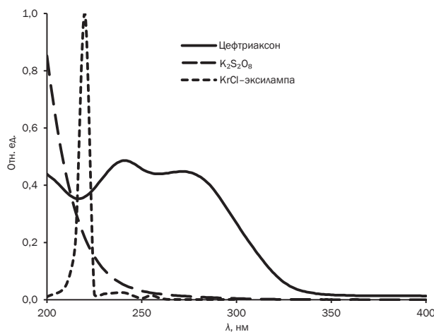
Рис. 1. Спектры поглощения водных растворов цефтриаксона, персульфата калия и спектр излучения КrCl-эксилампы
