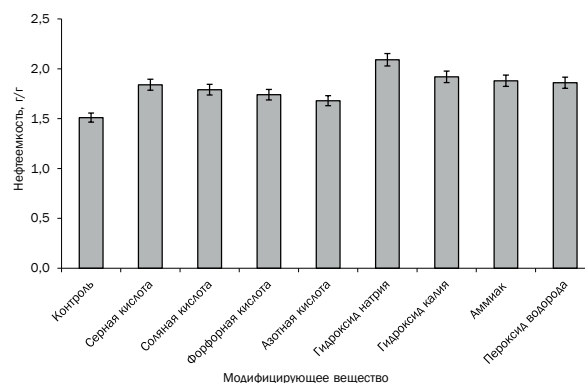
Рис. 1. Зависимость нефтеемкости отработанного кизельгура от вещества, применяемого для его модификации
