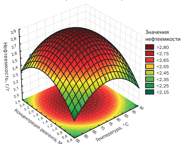
Рис. 5. Поверхность отклика зависимости нефтеемкости отработанного кизельгура от концентрации модифицирующего реагента и температуры проведения процесса модификации
