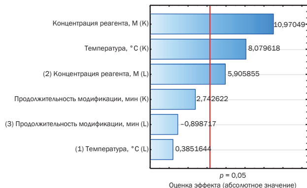
Рис. 9. Карта Парето стандартизованных эффектов
