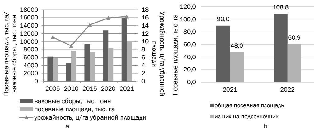
Рис. 2. Корреляция показателей валовых сборов, посевных площадей и урожайности подсолнечника в России в 2001–2021 гг. 1 (а); динамика роста посевных площадей в Республике Адыгея в 2021–2022 гг. 2 (б)
